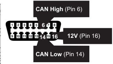
OBD-II connector Connecteur OBD-II
