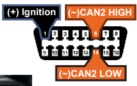
② OBD-II connector Connecteur OBD-II
