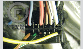
① Back view - Black 12-pin Immobilizer connector, at Ignition barrel. Vue de dos - Connecteur Noir d'immobilisateur, 12-pins, au barillet d'ignition.
