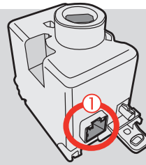
① Back view - Black 12-pin Immobilizer connector, at Ignition barrel. Vue de dos - Connecteur Noir d'immobilisateur, 12-pins, au barillet d'ignition.
