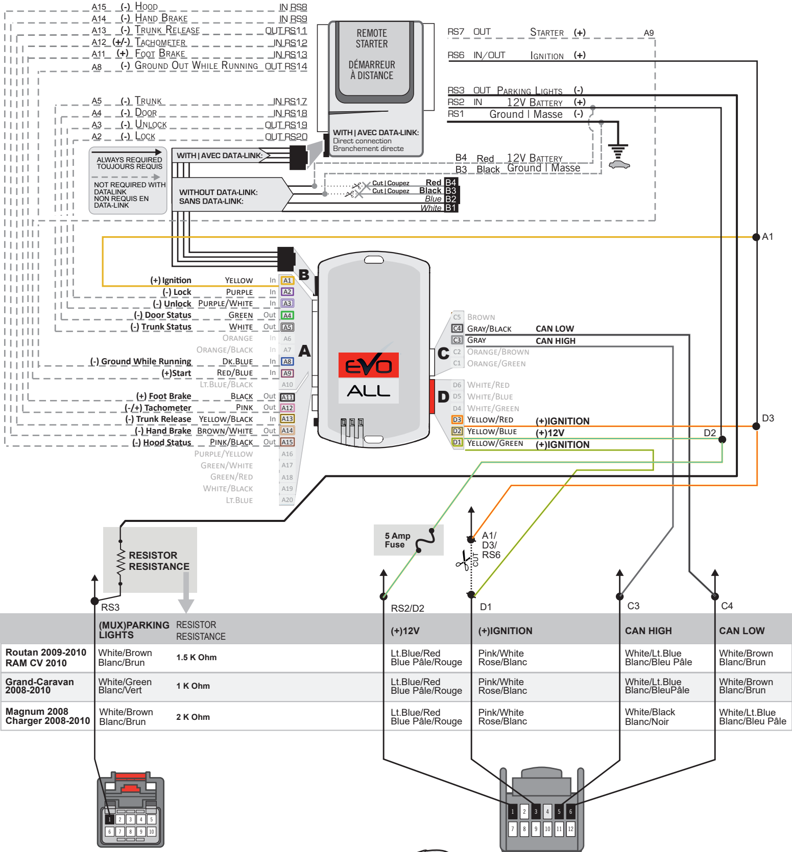
1 Back view - Black 12-pin Immobilizer connector, at Ignition barrel. Vue de dos - Connecteur Noir d'immobilisateur, 12-pins, au barillet d'ignition.
