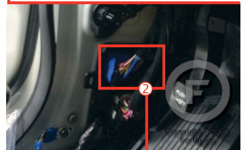
2 Driver kick panel. Panneau latéral côté conducteur.
