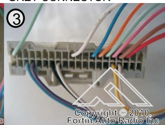
CONNECTEUR GRIS
