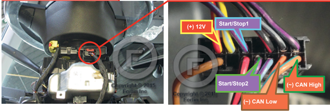
③ Under the steering column Sous la colonne de direction
