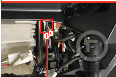
①C ECU, behind glove box ECU, derrière le coffre à gant
