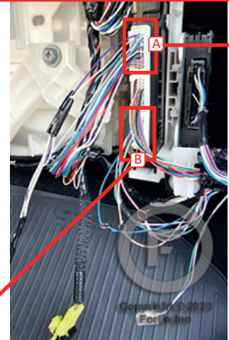
①C Certification ECU behind glove box ECU certification derrière le coffre à gants
