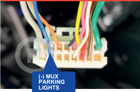
2 A Parking lights switch commutateur des feux de stationnement
