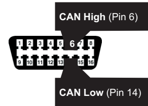
OBD-II connector Connecteur OBD-II
