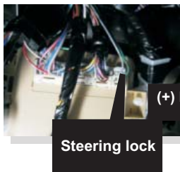
Back of BCM Au dos du BCM
