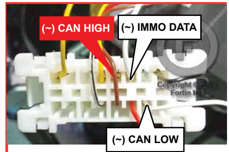
② OBD-II connector Connecteur OBD-II
